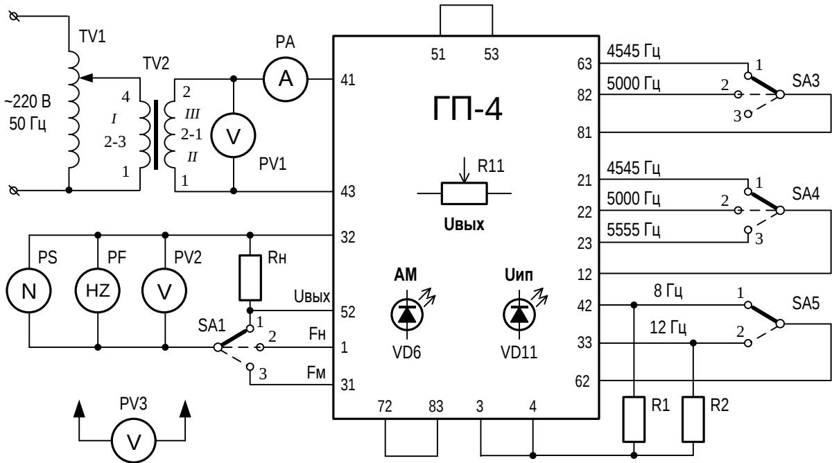
Рисунок Б.1 Схема проверки генератора ГП-4
